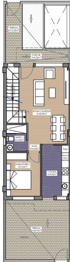
PLANTA BAJA
